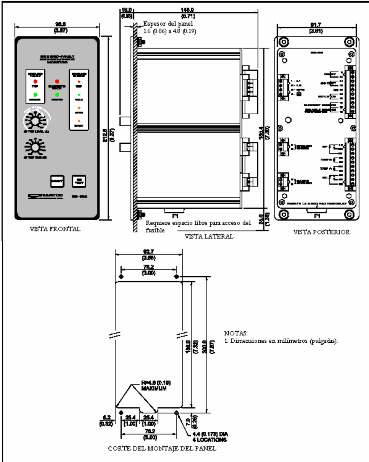
FIGURA 2. Detalles de trazado y montaje del panel de SE-134.
