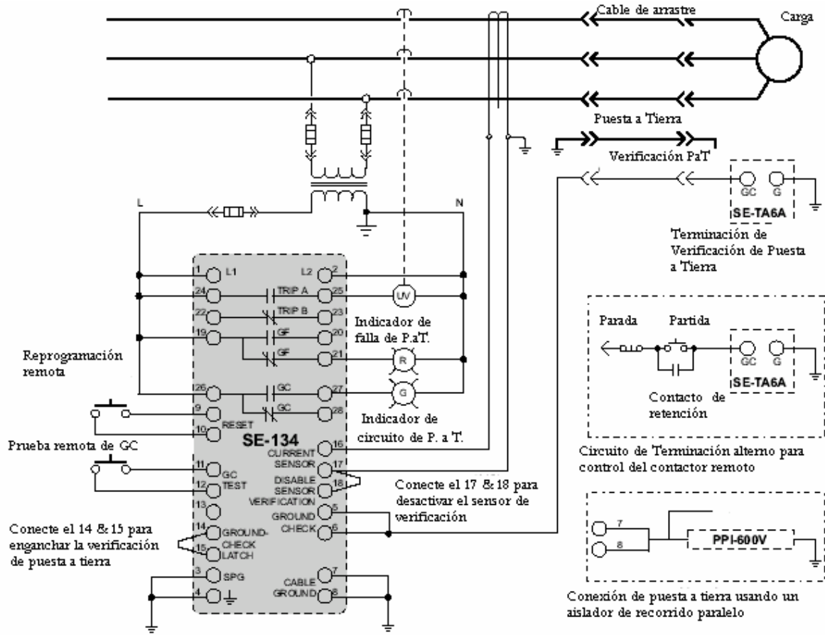
FIGURA 1. SE-134 Aplicación Típica
