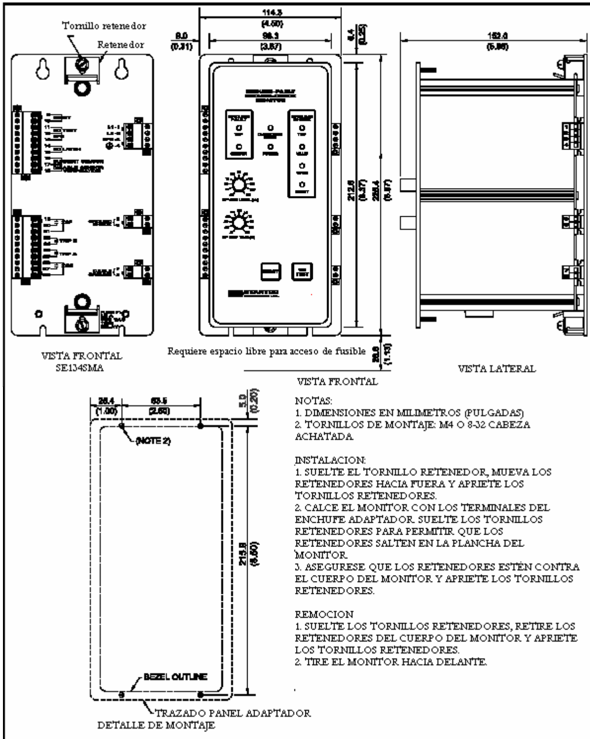
FIGURA 3. Detalles del Trazado y Montaje de Superficie del SE-134.
