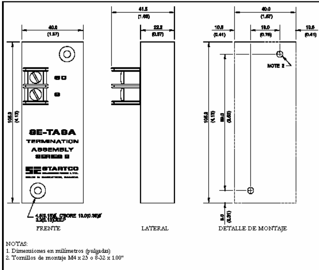
FIGURA 5. Conjunto de Terminación SE-TA6A.
