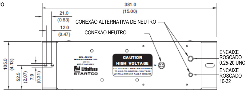
VISÃO SUPERIOR
