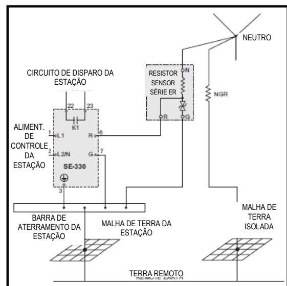
Figura 15 – Conexão Simplificada de Terra Isolado
