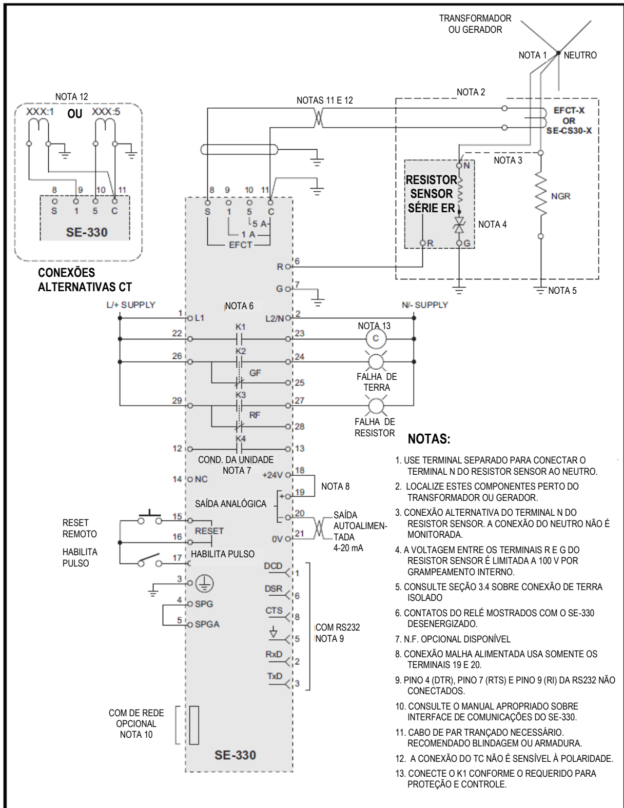
Figura 3 – SE-330 – Diagrama de Conexões
