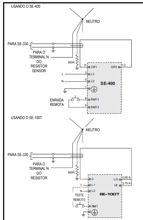
Figura 17 – Circuitos de Teste de Falta à Terra.
