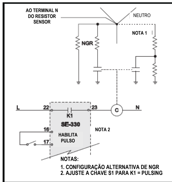
Figura 16 - Conexão Simplificada do Sistema de Pulsos
