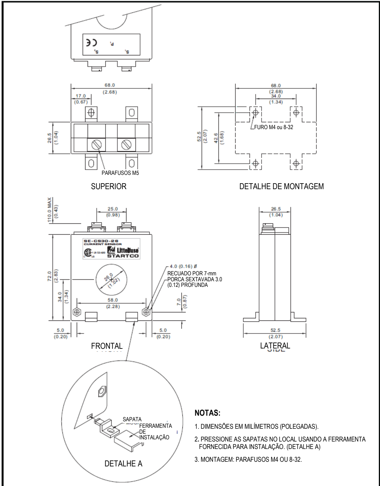
Figura 13 – EFCT-26 e SE-CS30-26 – Sensores Sensíveis de Corrente de Falta à Terra
