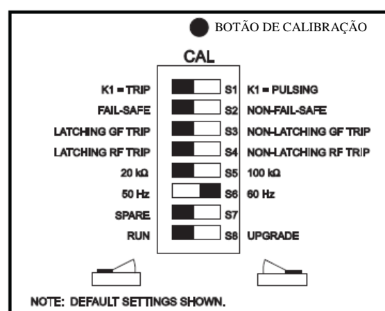
FIGURA 1 - Chaves de Configuração.
