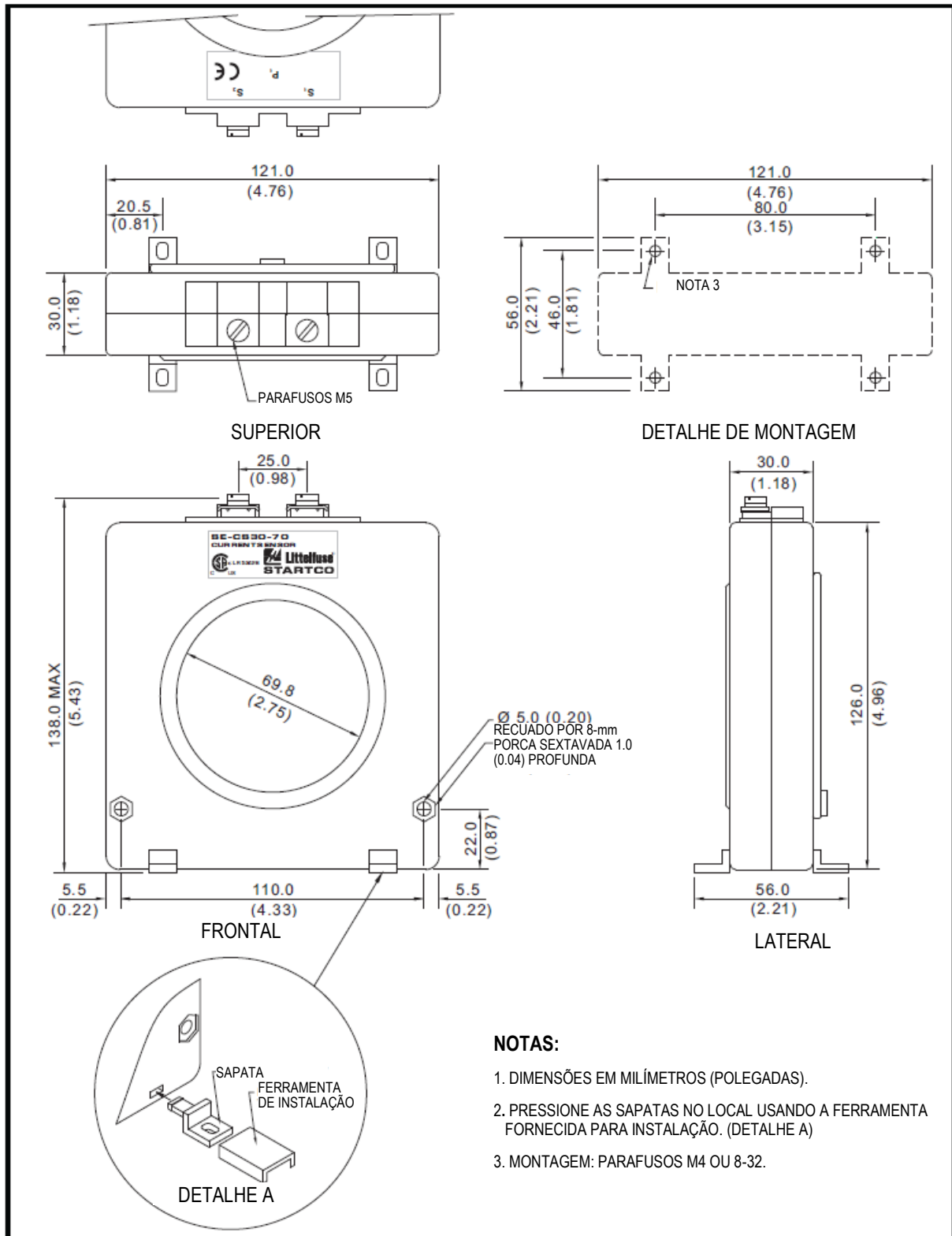
Figura 12 – SE-CS30-70 – Sensor Sensível de Corrente de Falta à Terra
