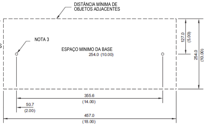
DETALHE DE MONTAGEM
