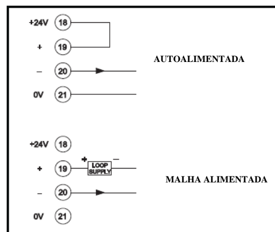
Figura 2. Conexões da Saída Analógica.
