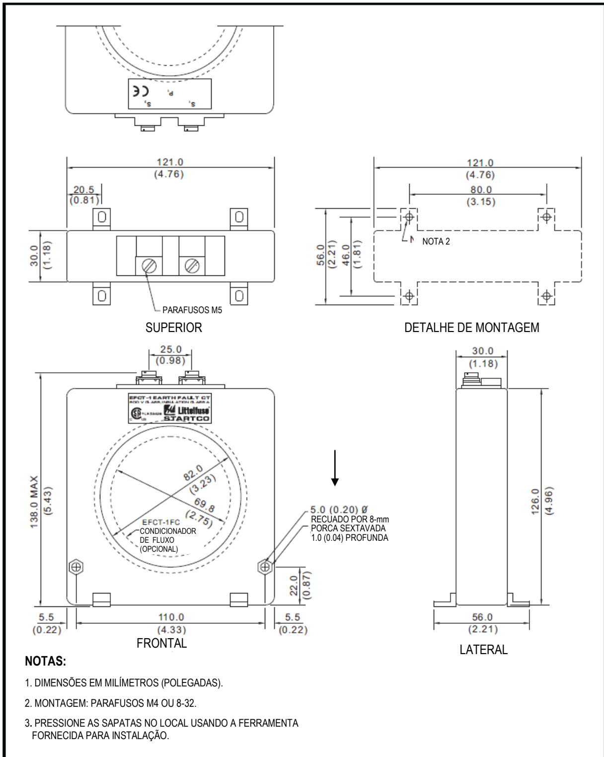
Figura 11 – EFCT-1 – Sensor Sensível de Corrente de Falta à Terra
